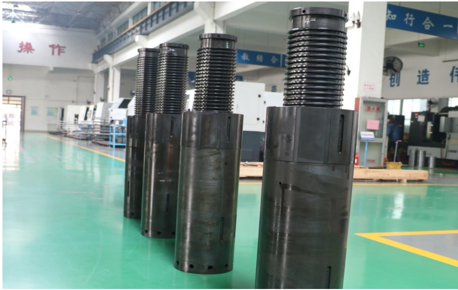
图 5-3 三峡用重载梯形丝杠副
